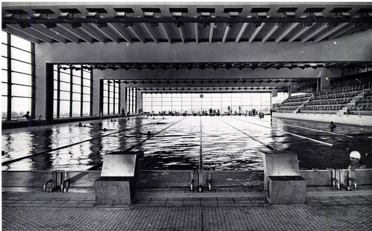
34. kép Balaton uszoda, Balatonfűzfő, Patonai Dénes MÉ 1982/6
