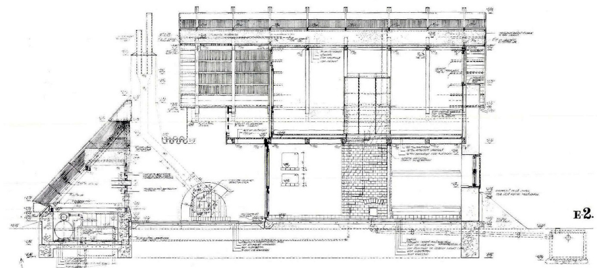
37.kép Ikernyaráló, Ábrahámhegy, Gulyás Zoltán, hosszmetset MÉ 1968/2
