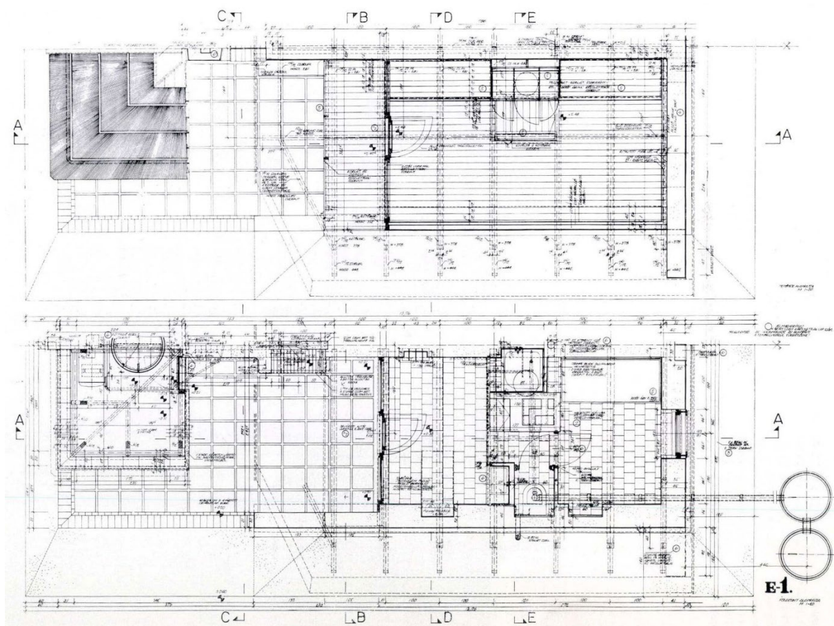
36.kép Ikernyaráló, Ábrahámhegy, Gulyás Zoltán, alaprajzok, MÉ 1968/2
